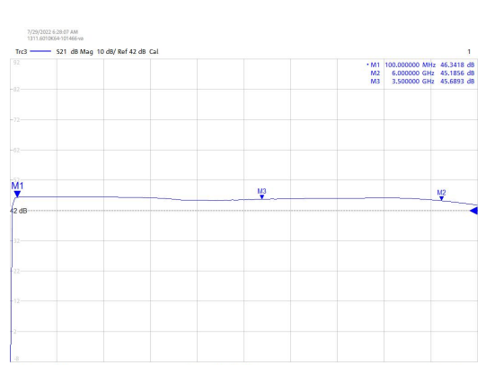
S21
